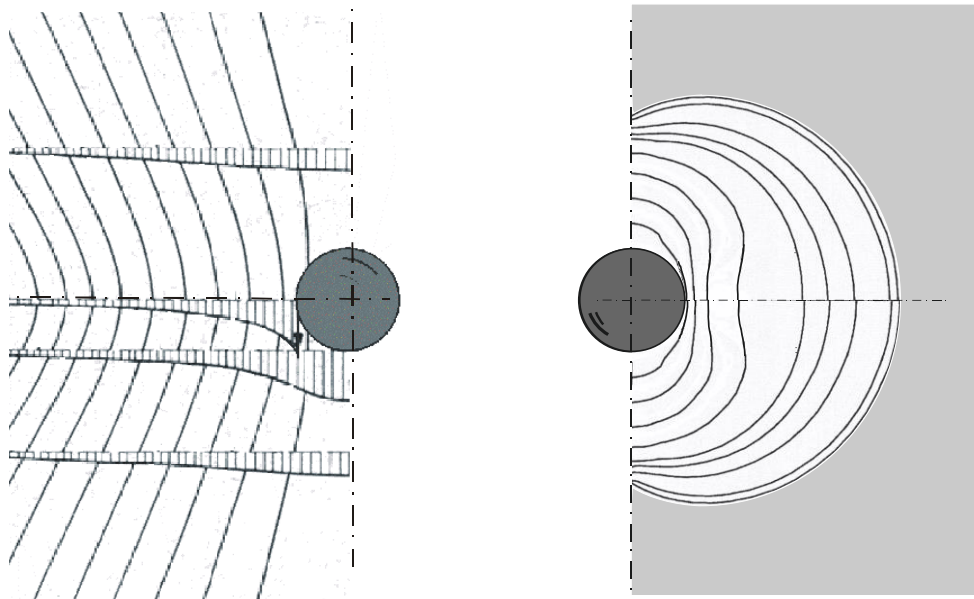
b.) BINGHAM-Fluid in Anlehnung an /4/
